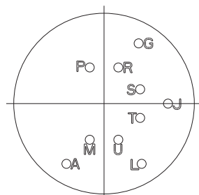
10-pos.
