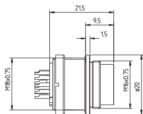
Lötanschluss
