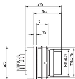
Lötanschluss
