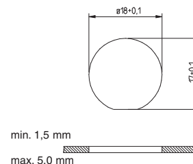
Einbaumaße
