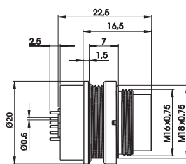
Einlötanschluss
