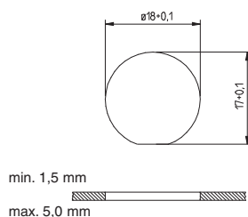
Einbaumaße
